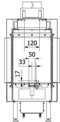
A-A (1 : 10)
