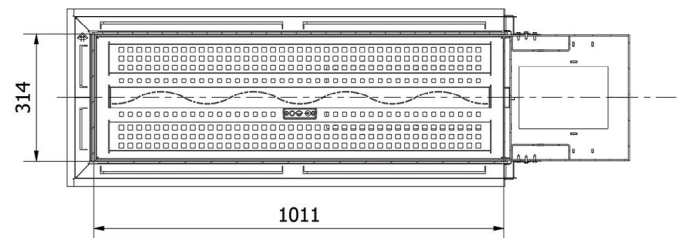
B-B (1 : 10)
